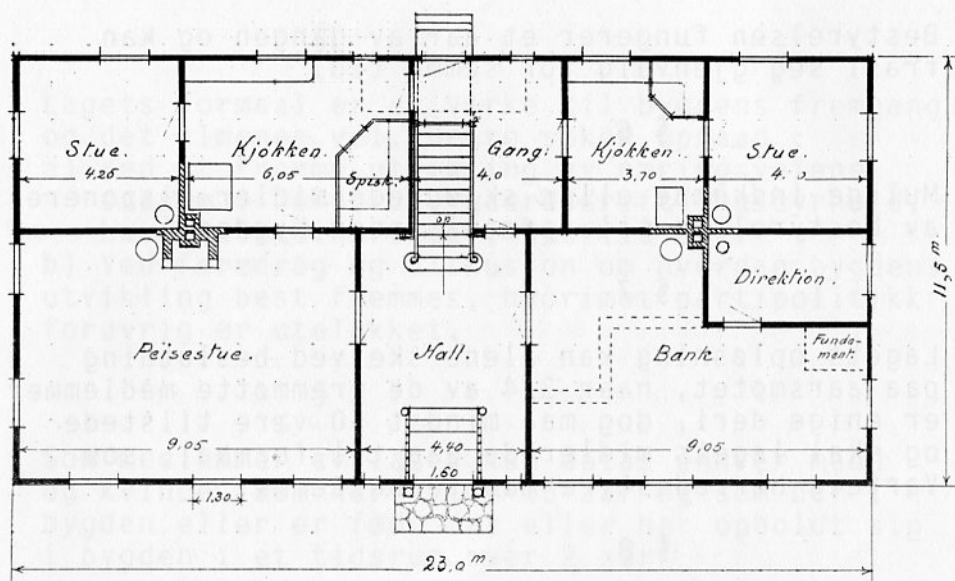
1 ste Etage.
